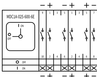
MDC1A 025-600-6 E IEC
