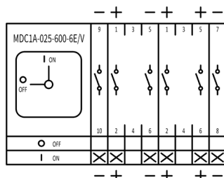
MDC1A 025-600-6 E/V UL
