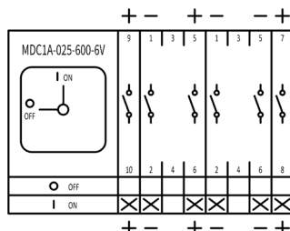
MDC1A 025-600-6 V IEC
